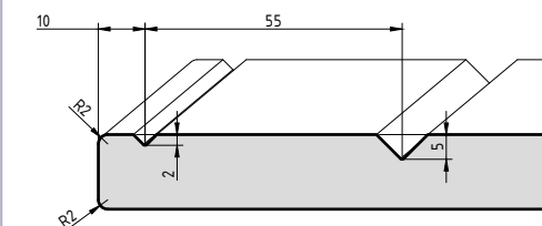
Чертеж разреза фрезеровки
